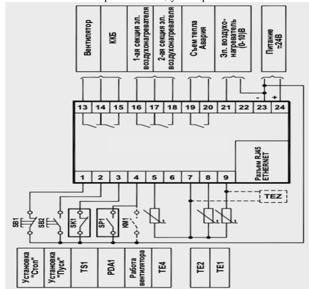
Схема 4. Электрический воздушонагреватель и ККБ.
