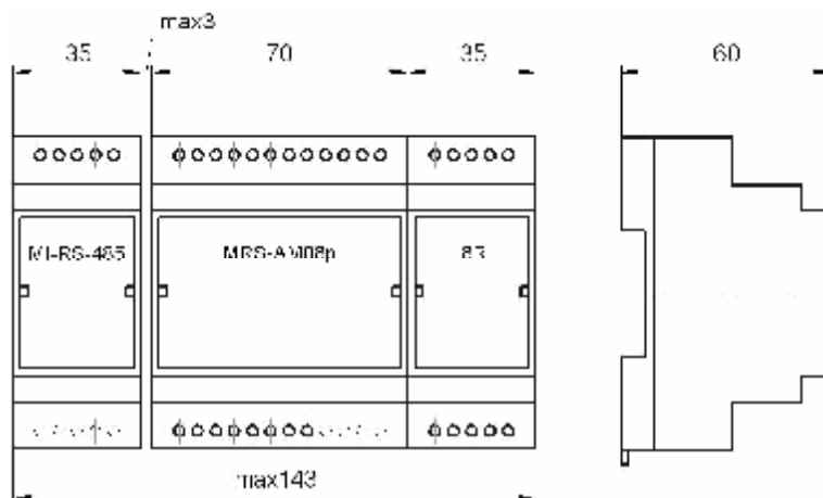
Рис. 1. Габаритные размеры контроллера.
