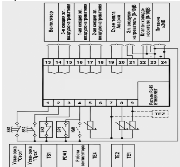
Схема 3. Электрический воздушонагреватель и водяной воздухоохладитель.
