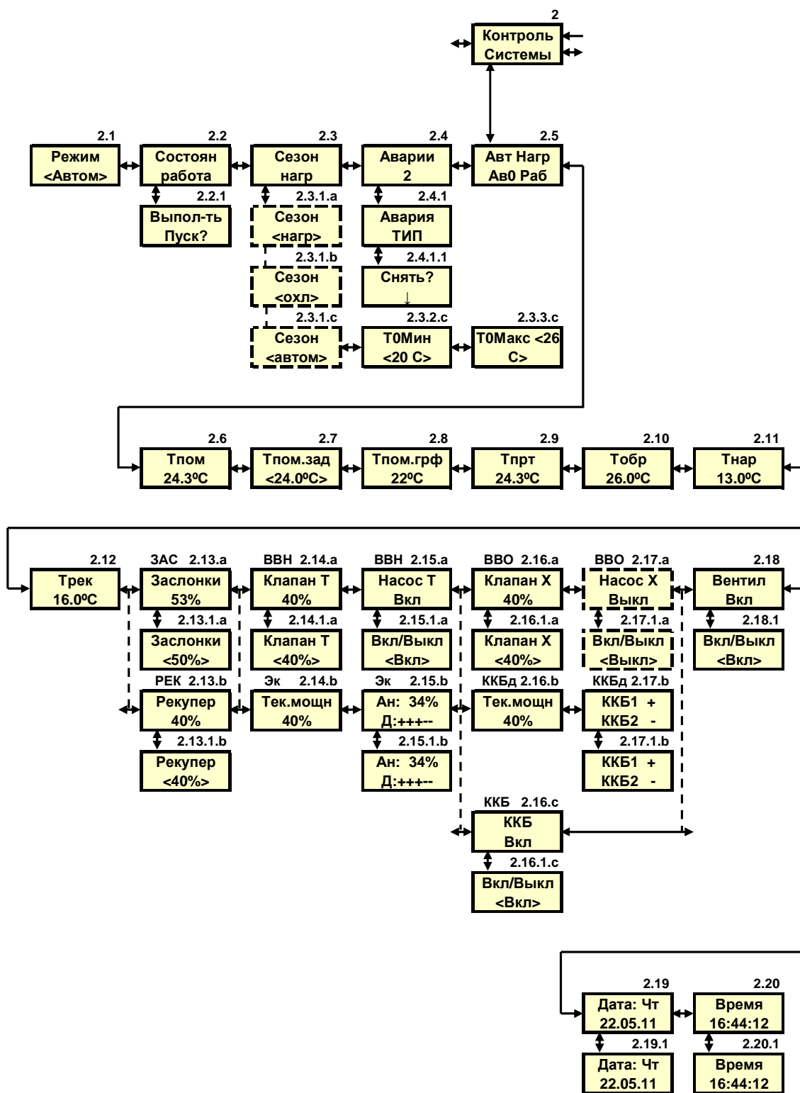
Рисунок 3. Ветка меню контроля системы.
