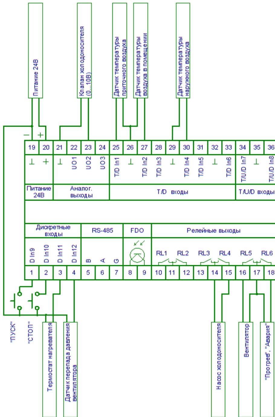
Рисунок 10. Подключение ВВО.
