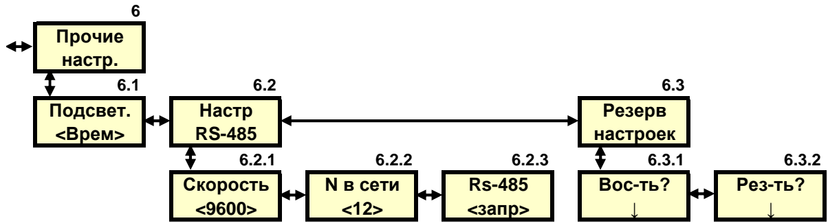
Рисунок 6. Ветка меню прочих настроек системы.
