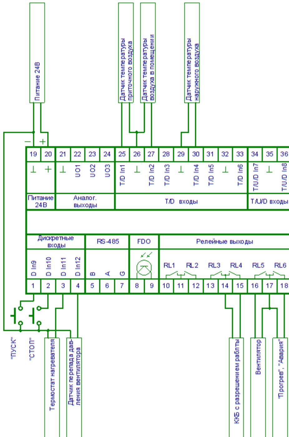
Рисунок 12. Подключение ККБ с разрешением работы.
