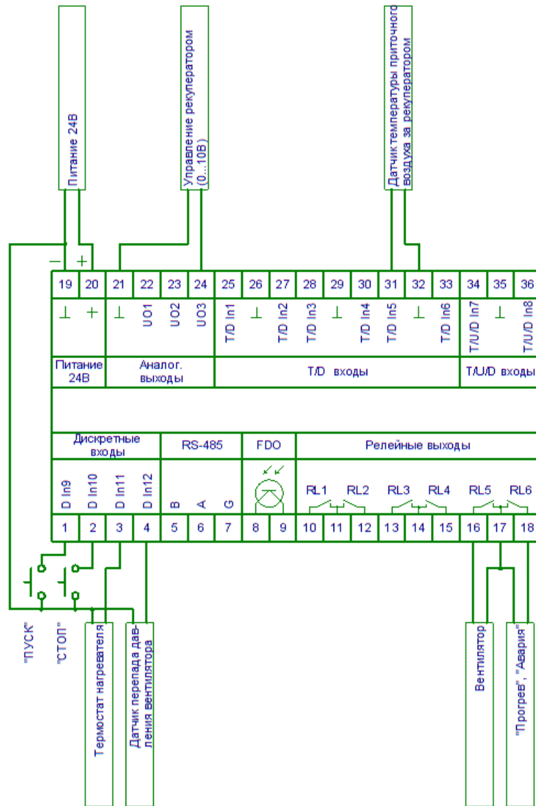
Рисунок 13. Подключение рекуператора.
