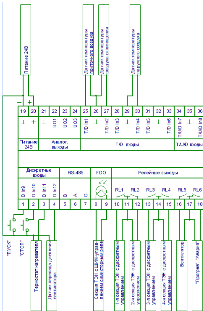
Рисунок 9. Подключение калорифера с ШИМ-управлением.
