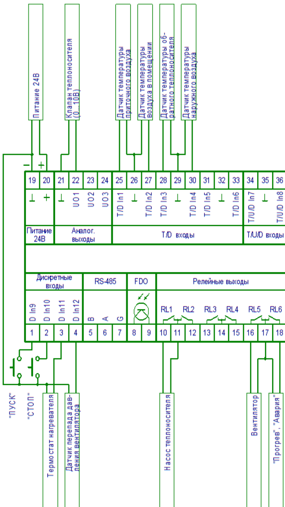
Рисунок 7. Подключение ВВН.
