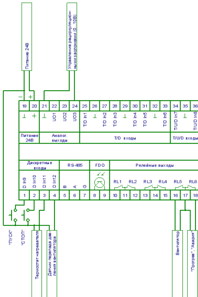
Рисунок 14. Подключение рециркуляционных заслонок.
