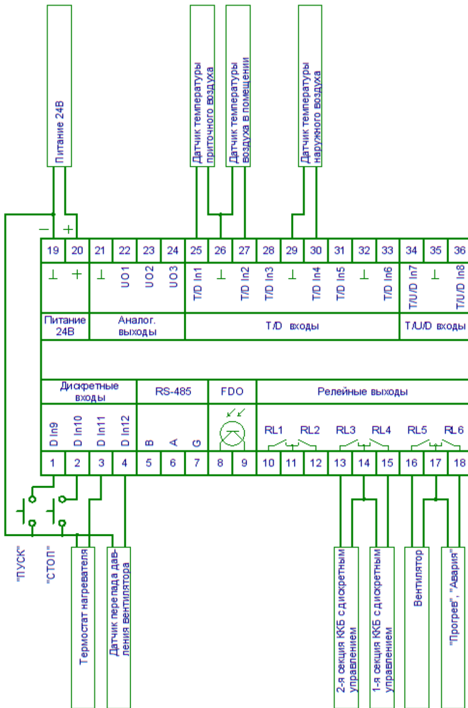
Рисунок 11. Подключение ККБ с дискретным управлением.
