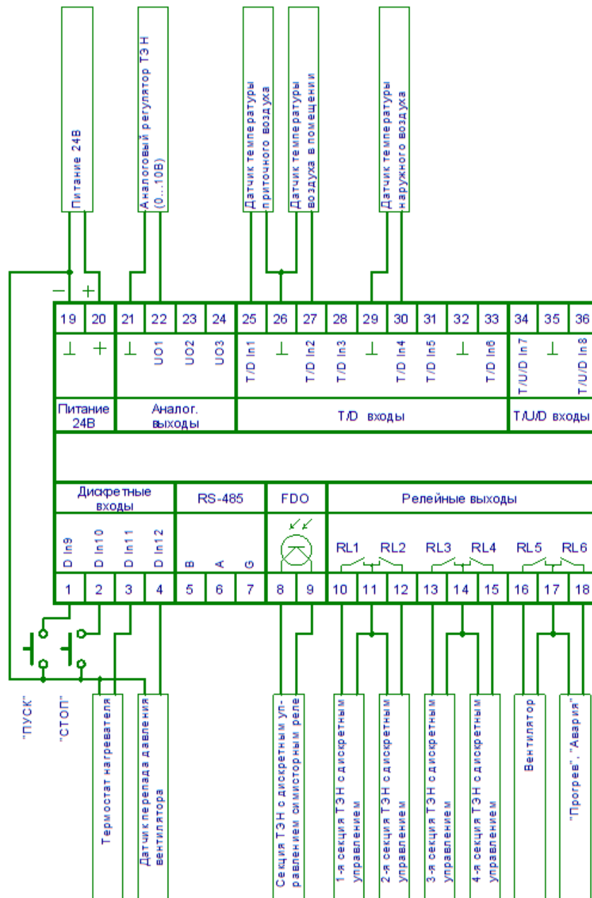
Рисунок 8. Подключение калорифера с аналоговым управлением.
