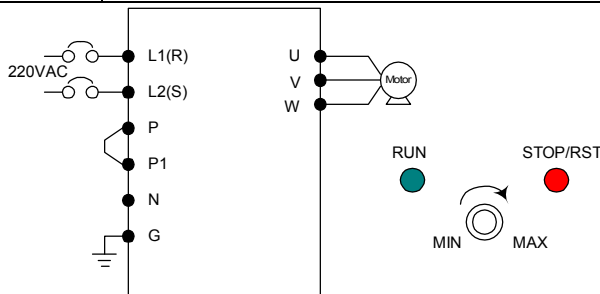
Схема подключения
