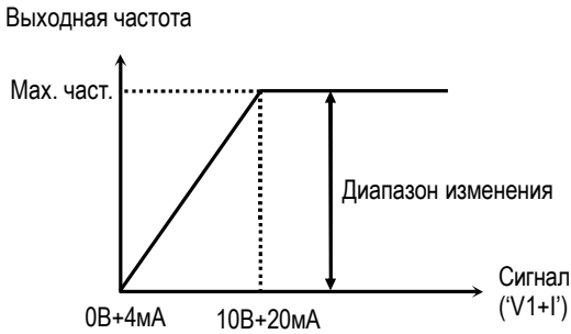
[Источник задания скорости: "V1+I"]
