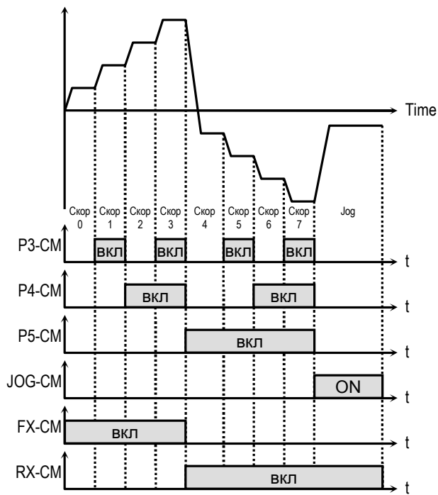
[Многоскоростной режим]
