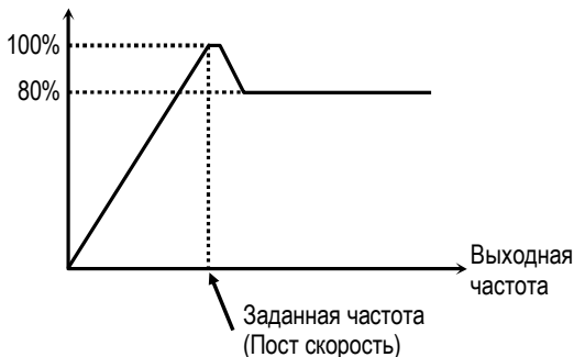
[Диаграмма работы при F40 = 20% ]
