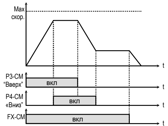
[Управление Вверх/Вниз]
