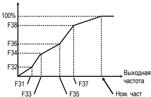
[Специальная U/F-характеристика]
