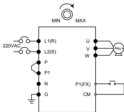
Схема подключения
