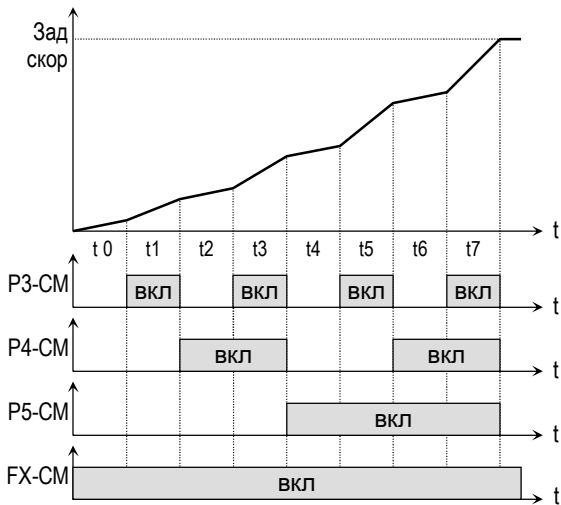
[Работа с различными временами разгона]
